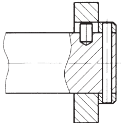
mit Stellring , Spannhülse und Verdrehsicherungsstift
