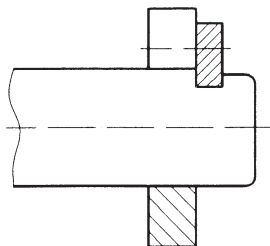
mit Achshalter
