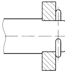
mit Splint
