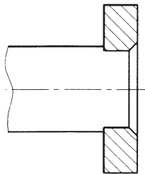
versenkt vernietet
