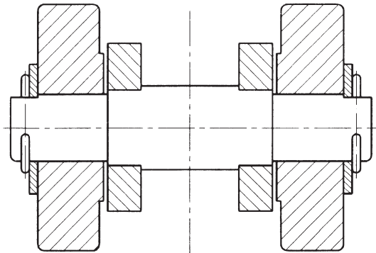
außenlaufende Rollen mit Scheibe und Splint
